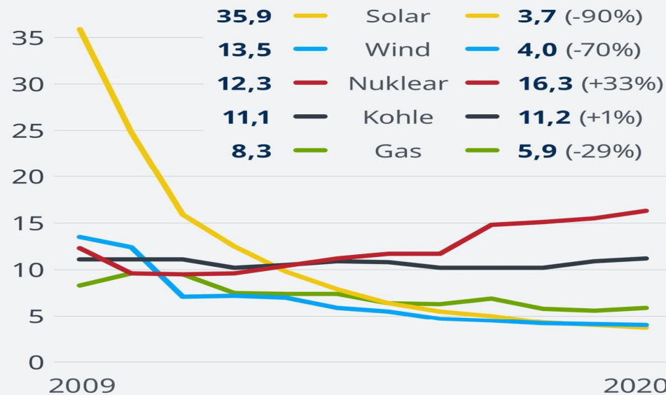
Solar- und Windstrom am günstigsten Erzeugungskosten in Dollar Cent/kWh
