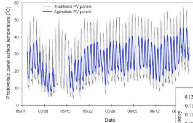
Temperatur der Module in FFPV und APV
